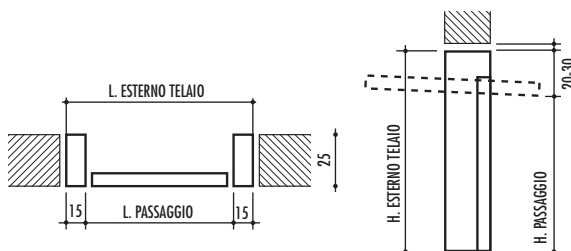
POSIZIONE IN LUCE
