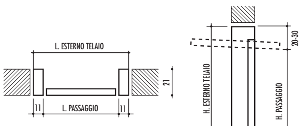
POSIZIONE IN LUCE
