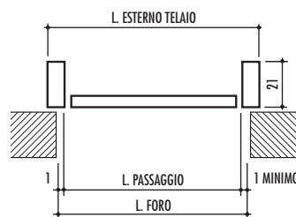
POSIZIONE OLTRE LUCE
