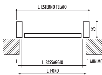
POSIZIONE OLTRE LUCE
