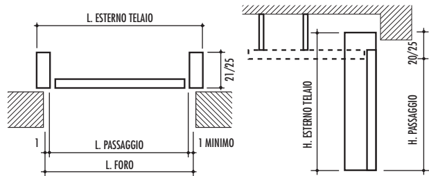
POSIZIONE OLTRE LUCE
