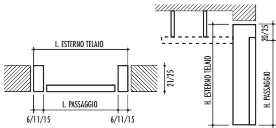
POSIZIONE IN LUCE
