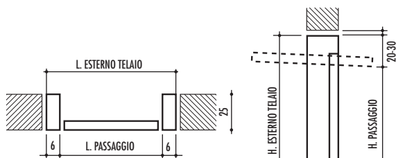
POSIZIONE IN LUCE
